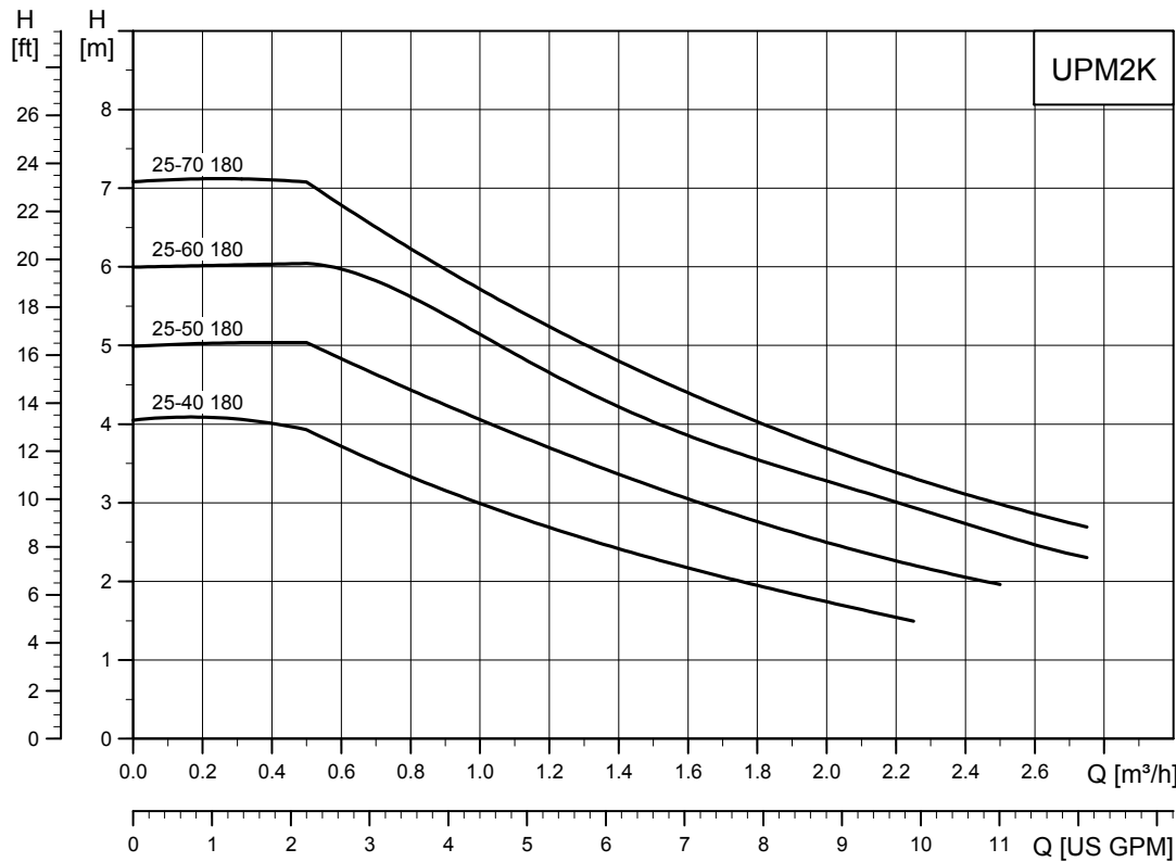
Fig. 3 UPM2K
